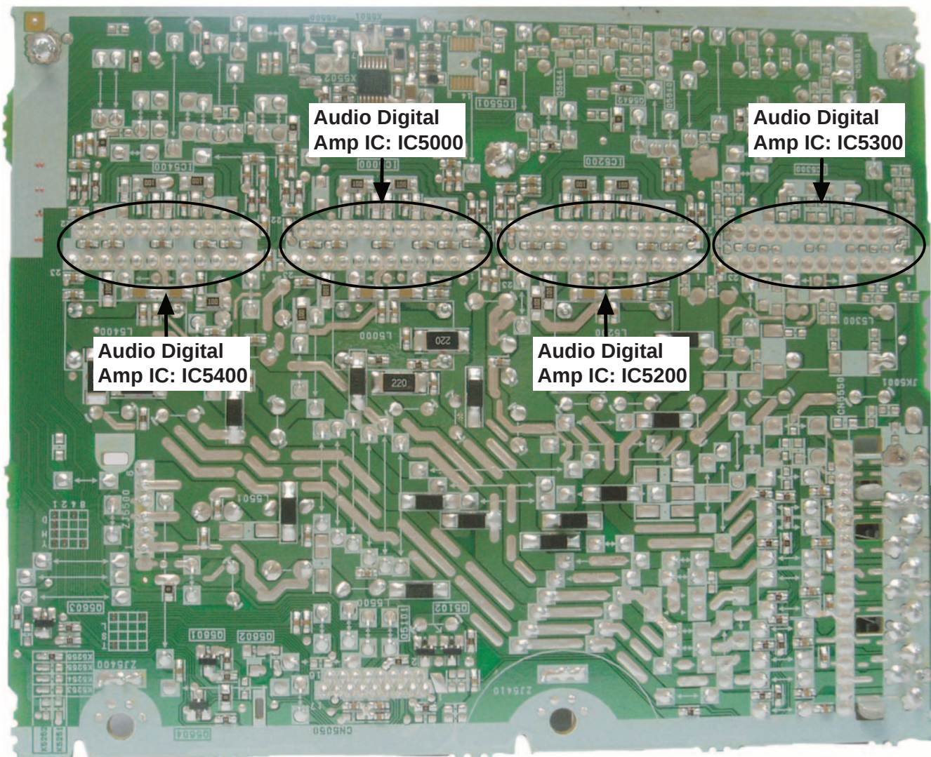
Fig. 3 D-Amp P.C.B.
