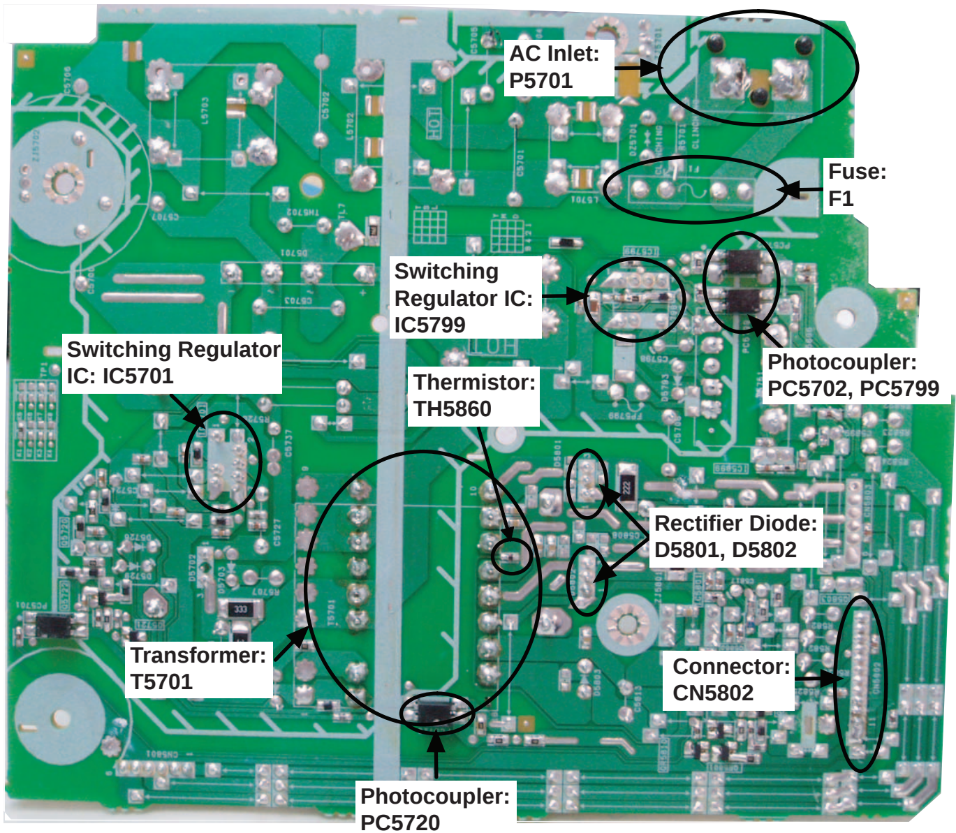
Fig. 1 SMPS P.C.B.
